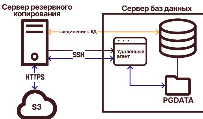
Рисунок G.1. Настройка pg_probackup с удалённым агентом и S3
