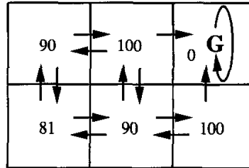
V^*(s) values
